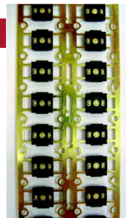
密冲压及二次成型模具
